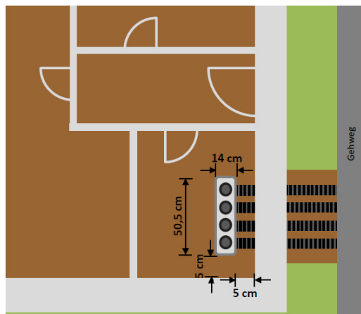
Abbildung 2: Draufsicht MSHE (nicht maßstäblich)
