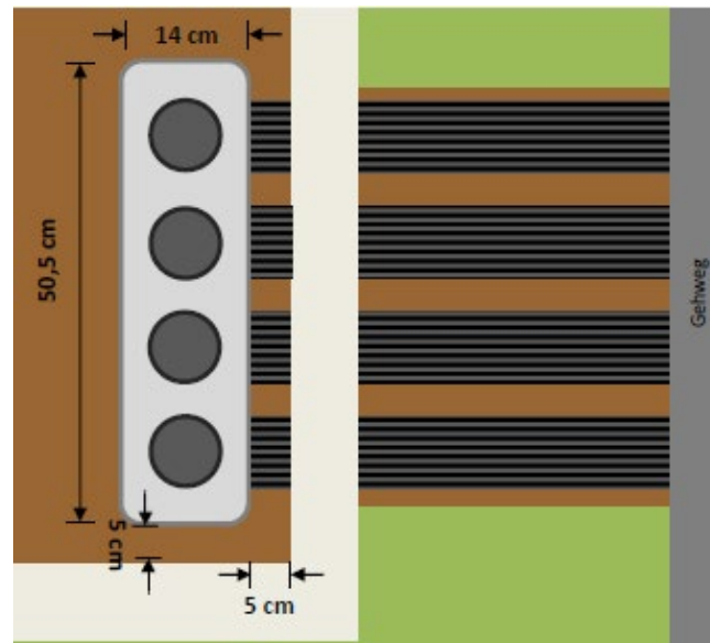
Abbildung 2 Draufsicht MSHE (nicht maßstäblich)
