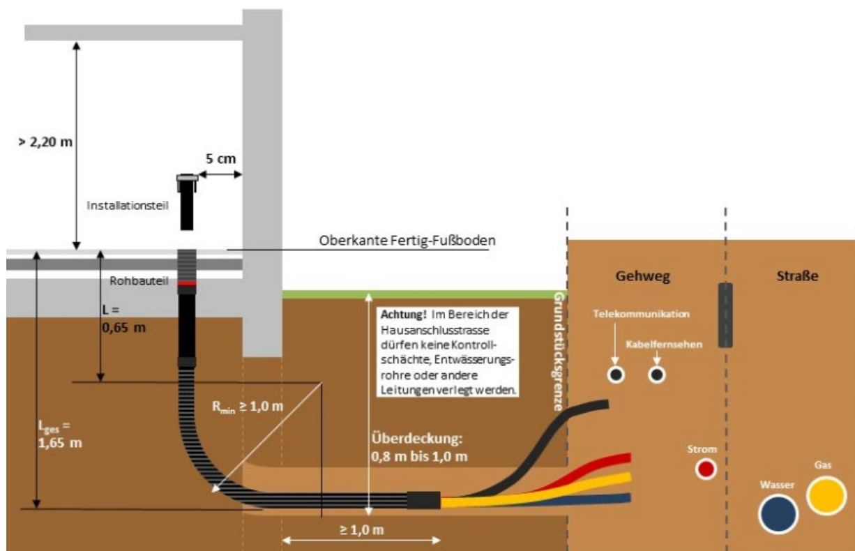
Abbildung 1 Seitenansicht MSHE (nicht maßstäblich)
