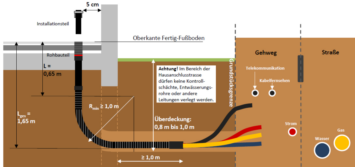
Abbildung 1: Seitenansicht MSHE (nicht maßstäblich)
